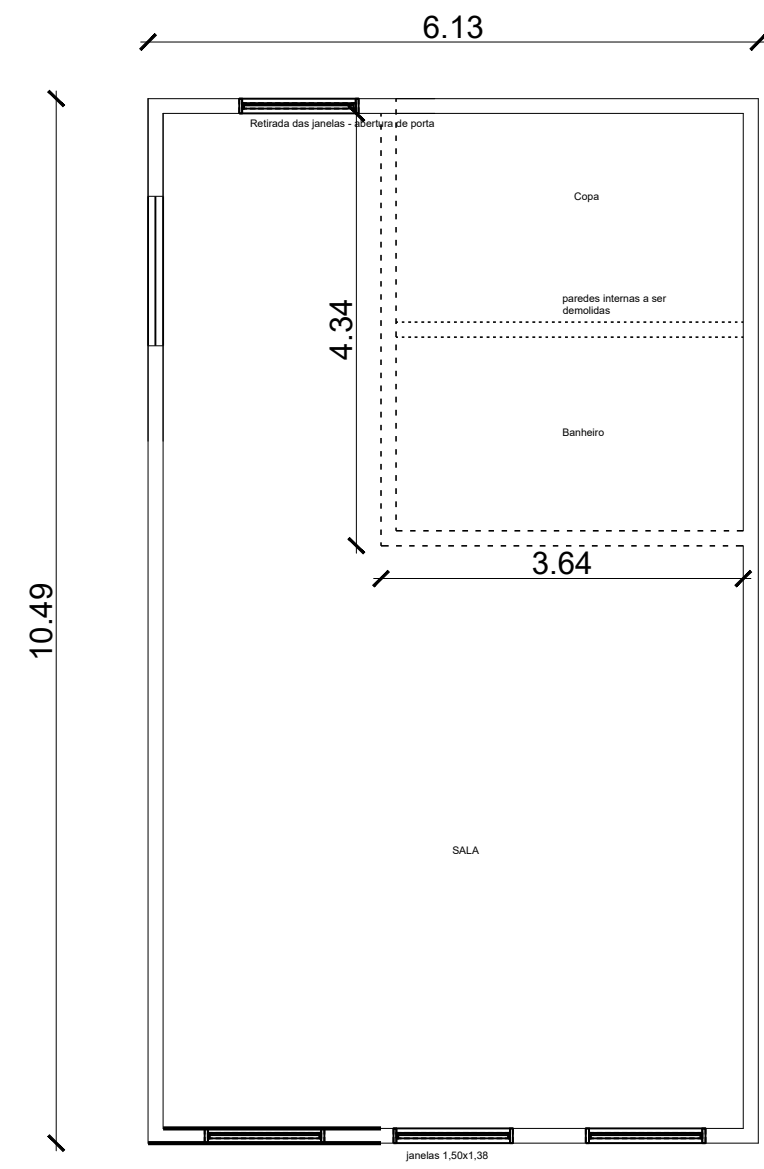
1 Planta Baixa situação atual Área à Construir: 64,30 m 2 Escala: 1/125
